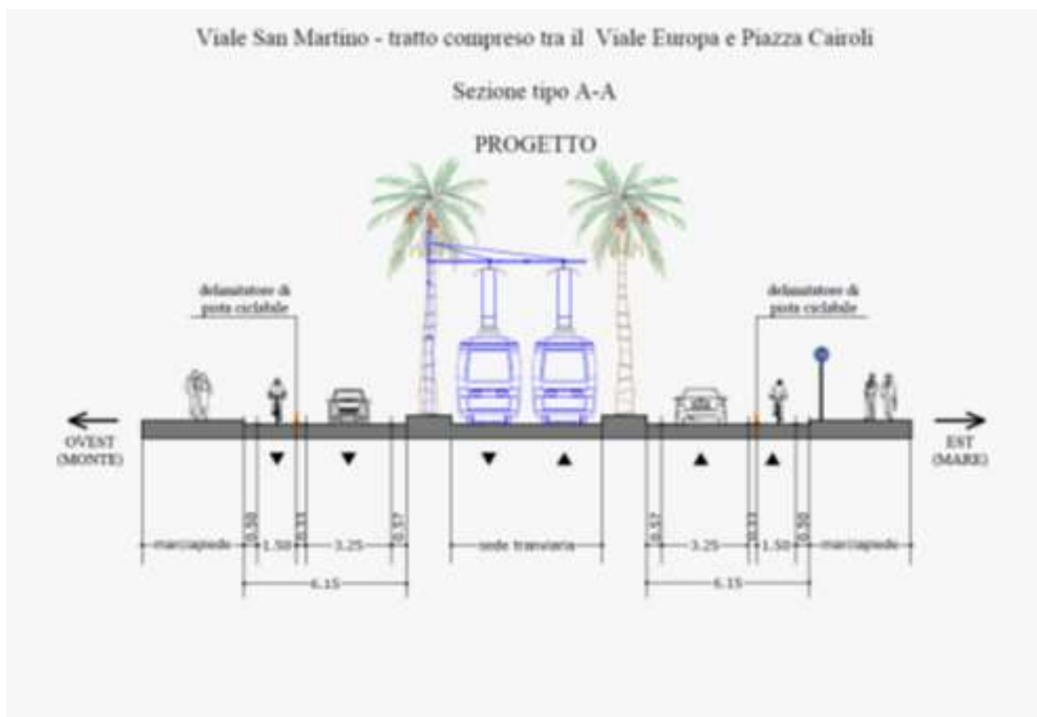
Fig. 2.d – Sezione tipo della pista ciclabile compresa nel tratto tra Viale Europa e Piazza Cairoli, come da progetto di “miglioramento della sicurezza ed estensione della pista ciclabile urbana del centro”.
