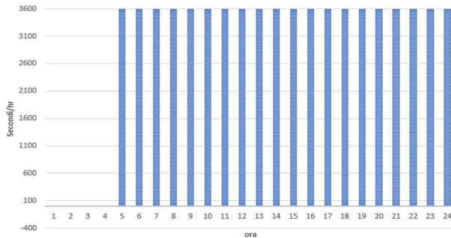
Fig. 4.I – Istogramma 24h caratteristico per la sorgente areale A4.
