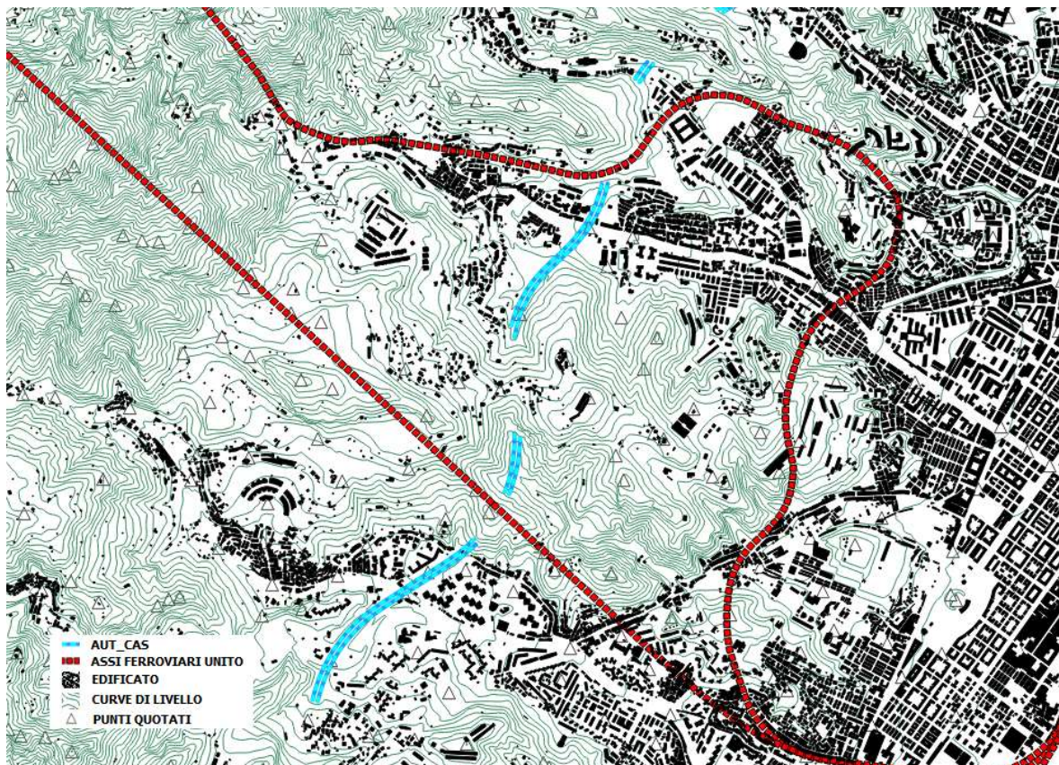
Fig. 4.a – Assi Autostradali, edificato, Linee Ferroviarie, Curve di Livello e Punti Quotati (CTR)
