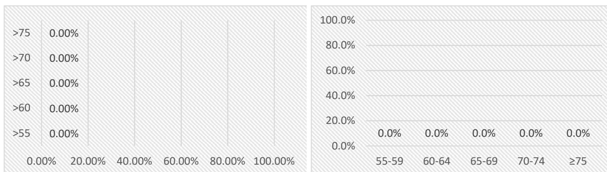
Fig. 7.ii – Major Railway Source: percentuali di strutture ospedaliere esposte e fasce Lden [dBA].
