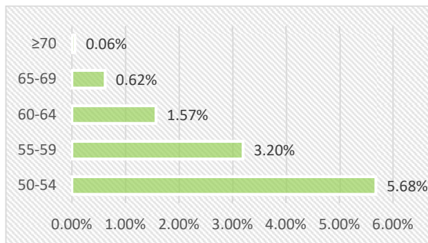
Fig. 7.aa – Major Road Source: percentuali di superficie territoriale esposta e fasce Ln [dBA].
