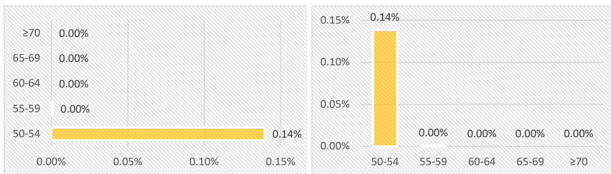
Fig. 7.ll – Major Railway Source: percentuali di popolazione residente esposta e fasce Ln [dBA].
