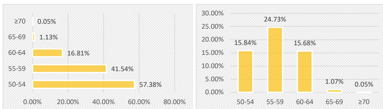
Fig. 7.r – Road Source: percentuali di popolazione residente esposta e fasce Ln [dBA].
