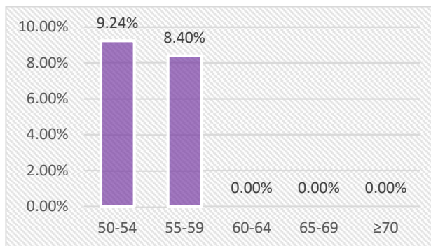
Fig. 7.cc – Major Road Source: percentuali di strutture scolastiche esposte e fasce Ln [dBA].
