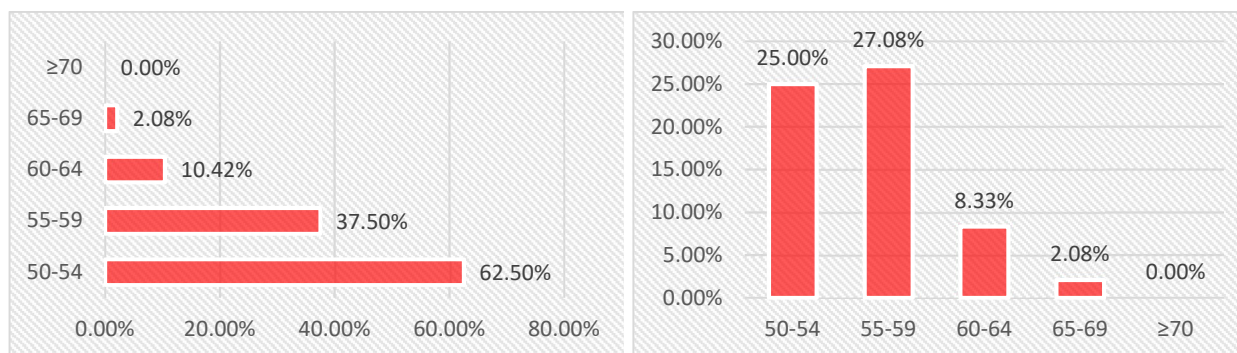
Fig. 7.t – Road Source: percentuali di strutture ospedaliere esposte e fasce Ln [dBA].
