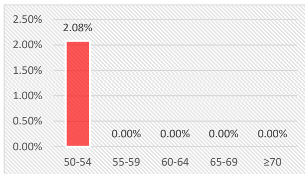
Fig. 7.dd – Major Road Source: percentuali di strutture ospedaliere esposte e fasce Ln [dBA].
