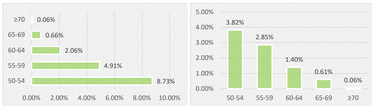
Fig. 7.q – Road Source: percentuali di superficie territoriale esposta e fasce Ln [dBA].
