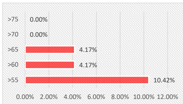
Fig. 7.ss – Industry Source: percentuali di strutture ospedaliere esposte e fasce Lden [dBA].
