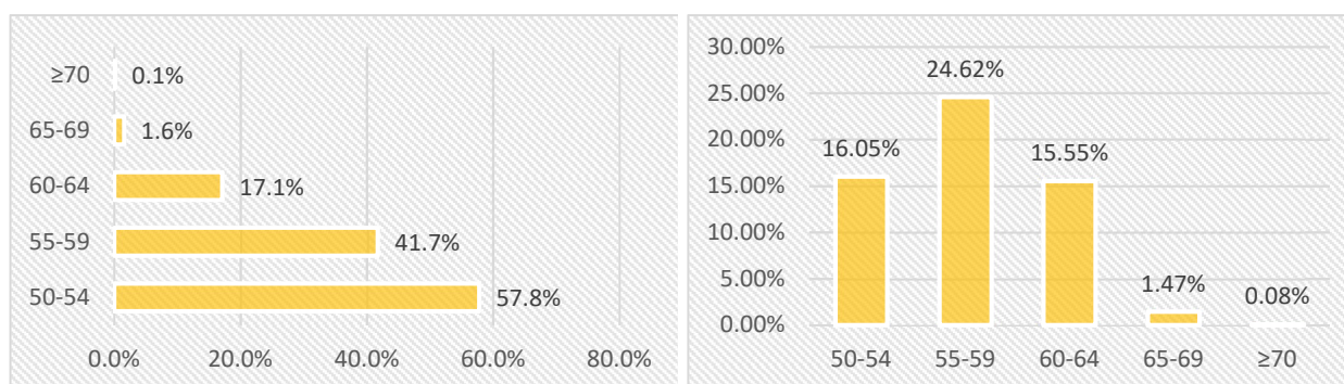
Fig. 7.h – Agglomeration Source: percentuali di popolazione residente esposta e fasce Ln [dBA].
