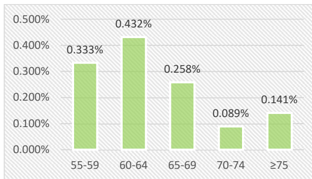
Fig. 7.pp – Industry Source: percentuali di superficie territoriale esposta e fasce Lden [dBA].
